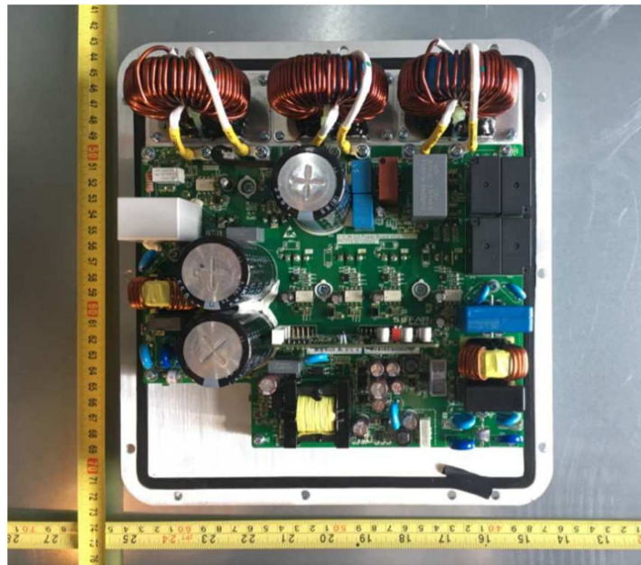
Figura 3, Visão interna Figure 3, Internal view
