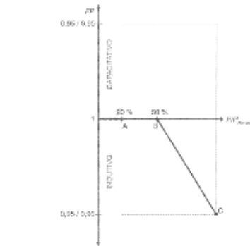
Figura 1 – Curva do FP em função da potência ativa de saída do inversor
